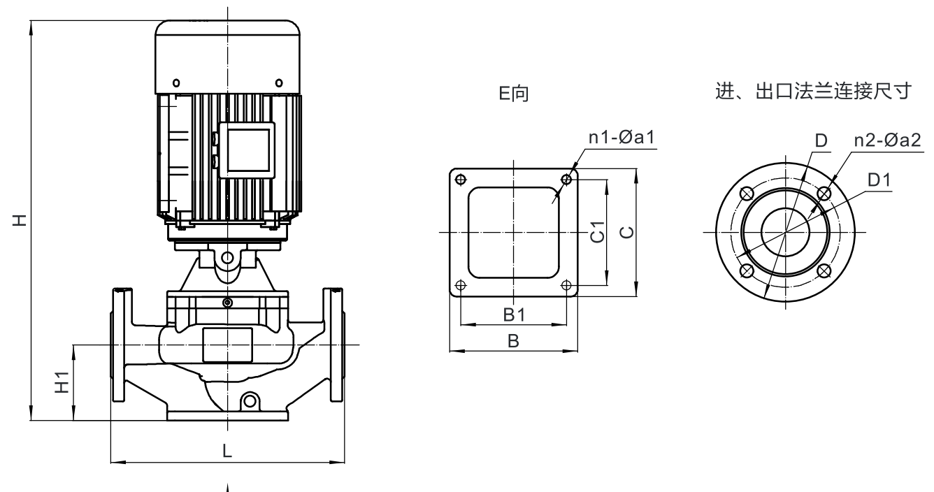
安装尺寸图
