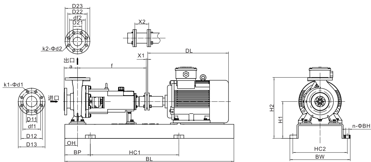
安装尺寸图
