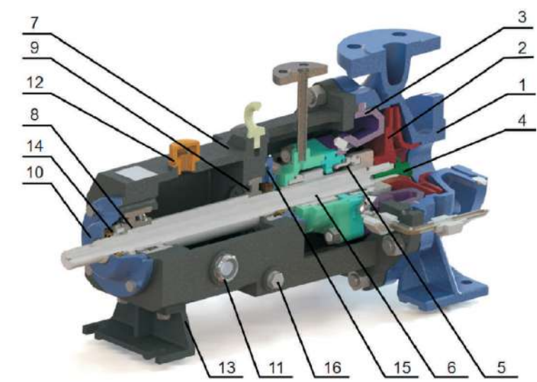
结构图
